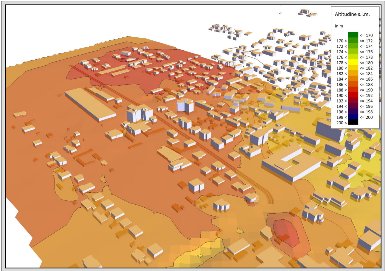
Figura 5 Discretizzazione del dominio di simulazione attorno al tratto di S.P. 231 di competenza del Comune di Parabiago
