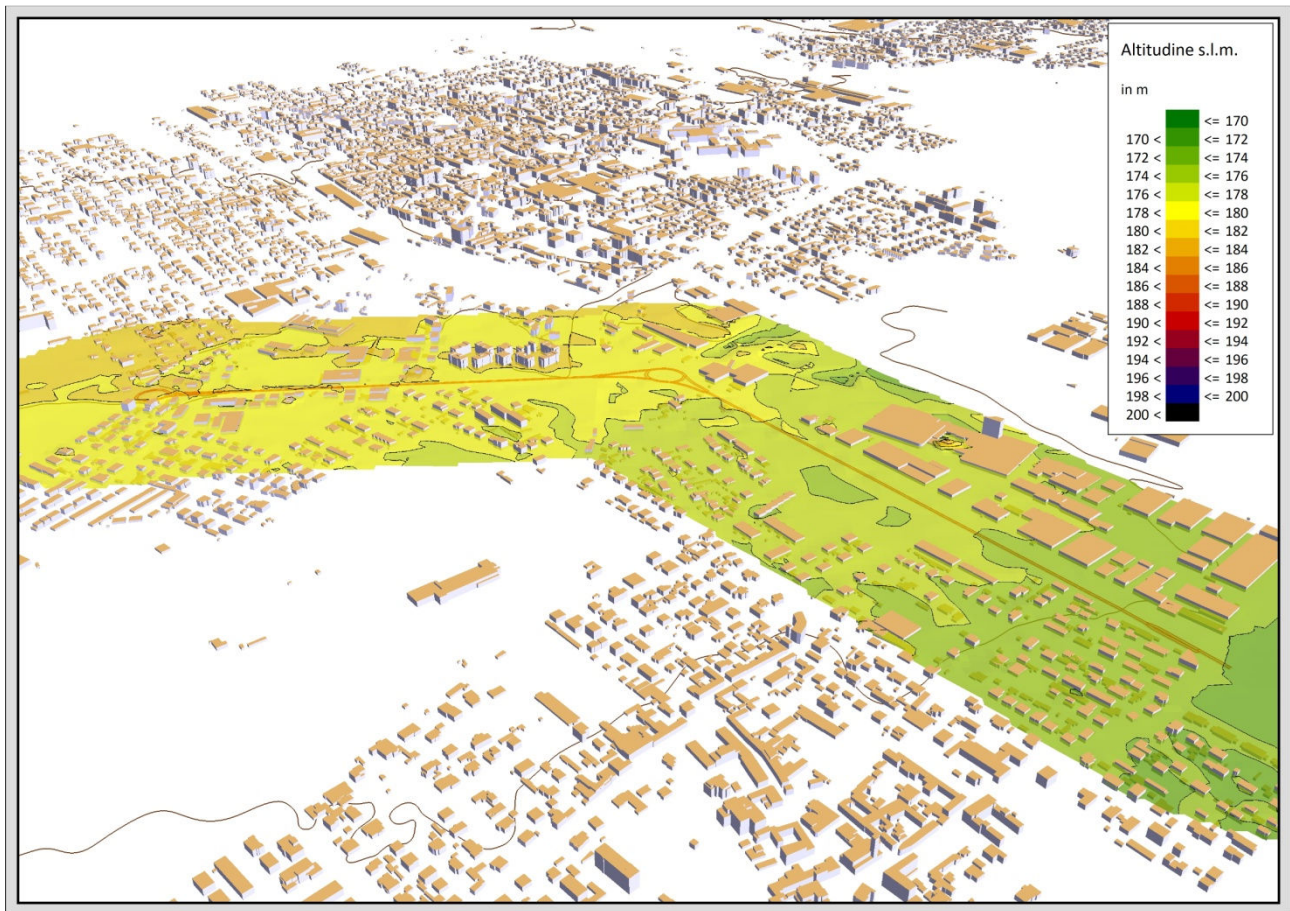
Figura 6 Discretizzazione del dominio di simulazione attorno al tratto di S.P. 109 di competenza del Comune di Parabiago
