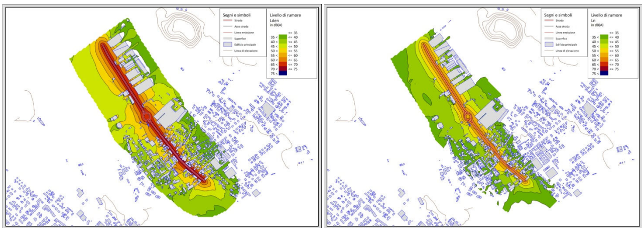
Figura 7 Mappe acustiche per i livelli L_{den} (a sinistra) e L_{night} (a destra) per il dominio di simulazione attorno al tratto di S.S. 33 del Sempione di competenza del Comune di Parabiago
