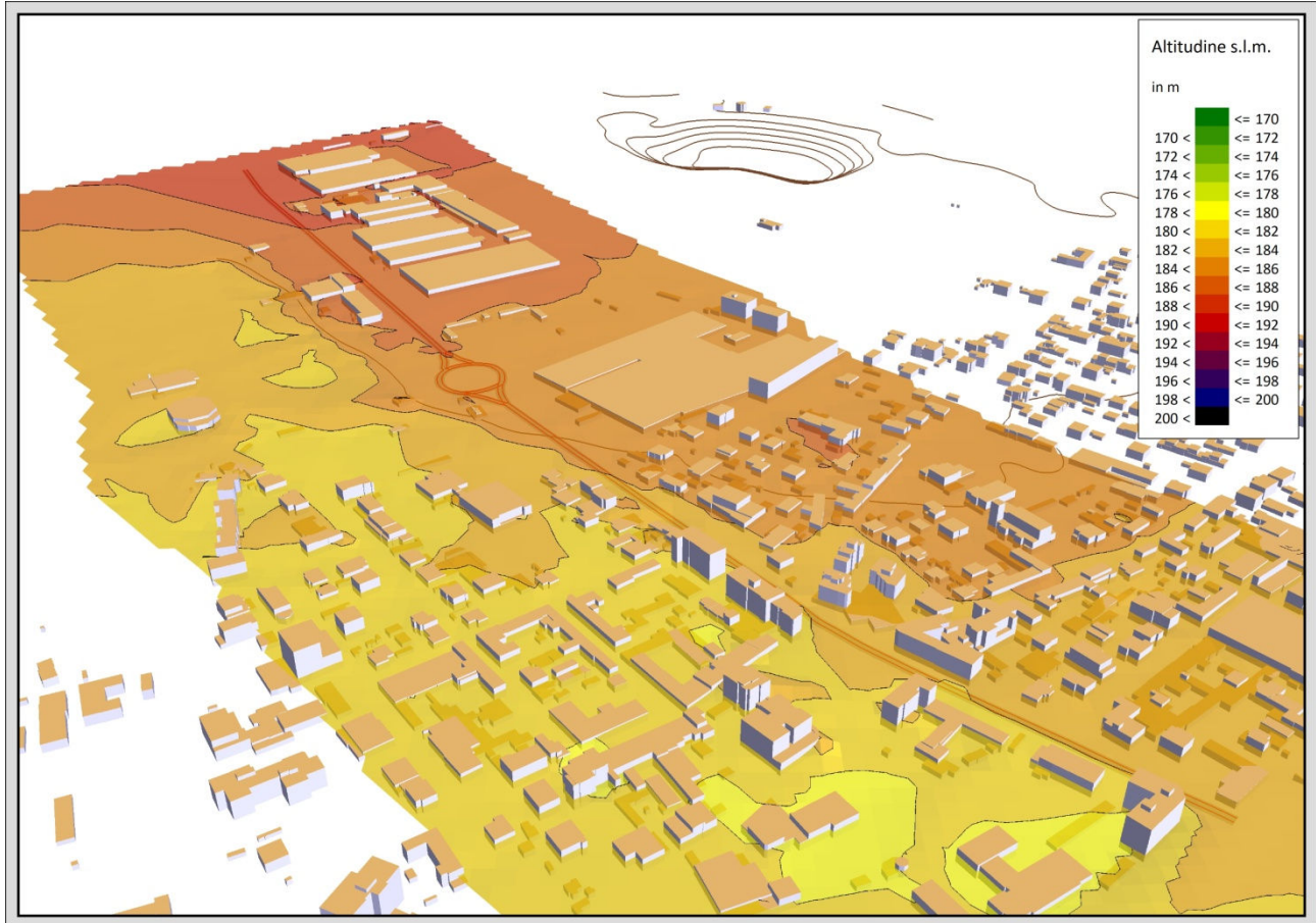
Figura 4 Discretizzazione del dominio di simulazione attorno al tratto di S.S. 33 del Sempione di competenza del Comune di Parabiago
