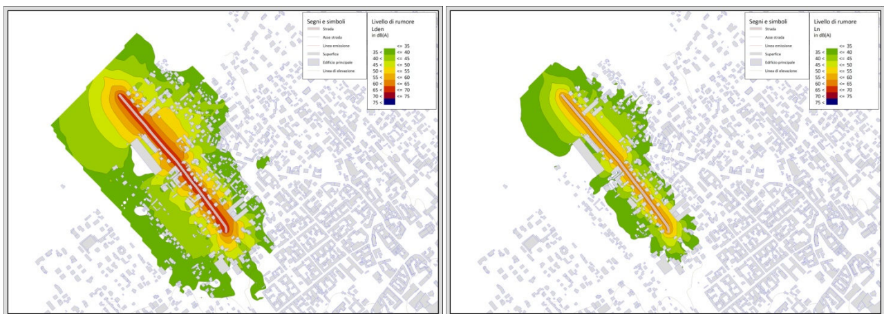
Figura 8 Mappe acustiche per i livelli L_{den} (a sinistra) e L_{night} (a destra) per il dominio di simulazione attorno al tratto di S.P. 231 di competenza del Comune di Parabiago
